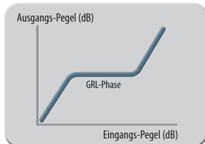
GRL Kennlinie
